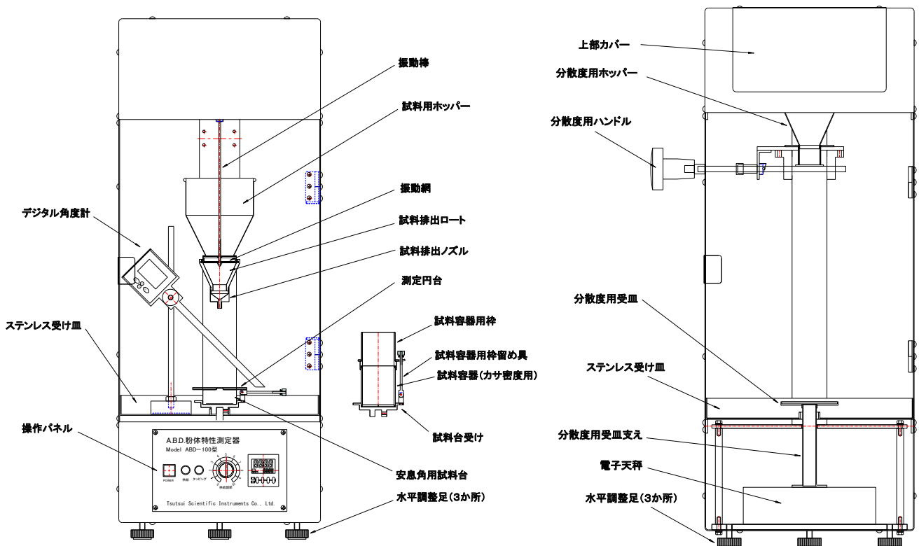
本体外観図
